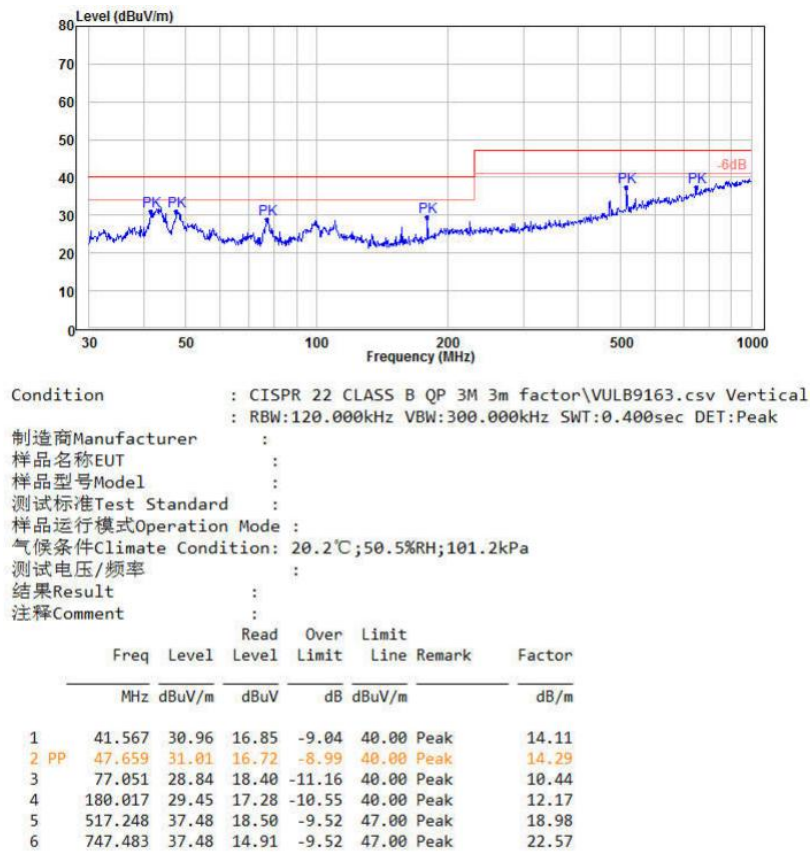
图 5-7 辐射测试垂直方向
