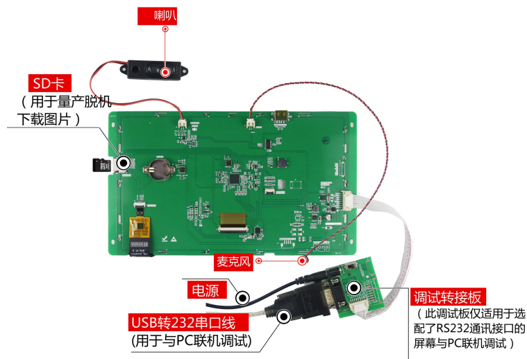
图 1-5 调试工具图
