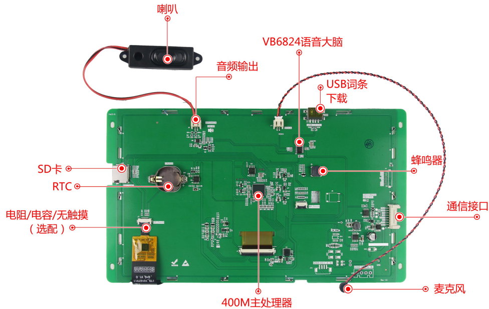
图 1-4 硬件配置图
